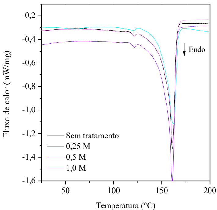
Figura 13 - Curvas de DSC das aparas de canudos tratadas e sem tratamento.
