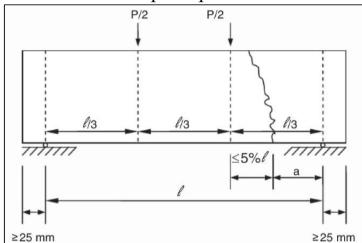
Figura 10 - Posicionamento da linha de ruptura fora do terço médio do corpo de prova.
