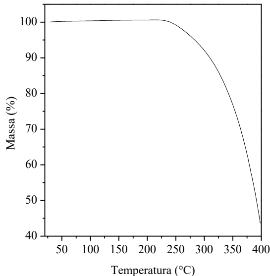
Figura 11 - Termogravimetria das aparas de canudos sem tratamento em atmosfera de ar sintético.
