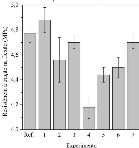
Figura 23 - Resistência à tração na flexão das diferentes composições.
