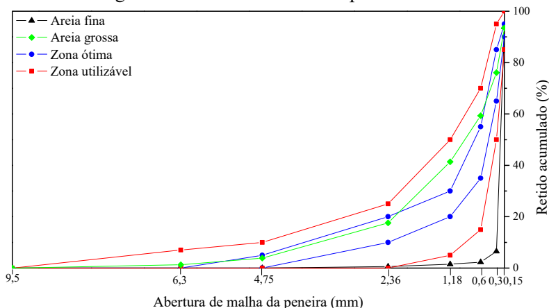
Figura 17 - Distribuição da composição granulométrica das areias fina e grossa e limites estabelecidos pela norma.
