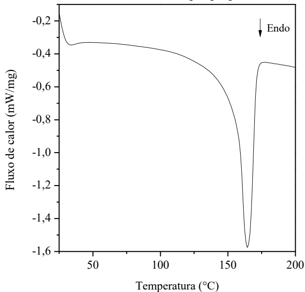
Figura 28 - Curva de DSC da fibra de polipropileno comercial.
