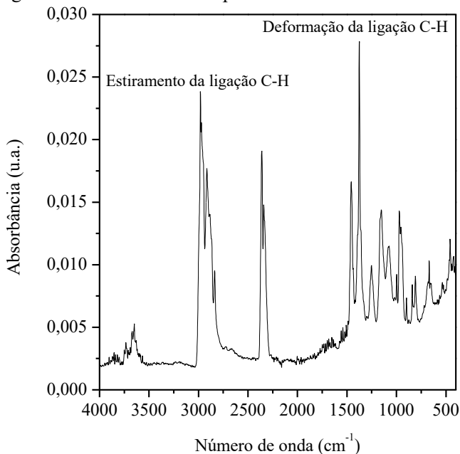
Figura 12 - FTIR/ATR das aparas de canudos descartáveis.
