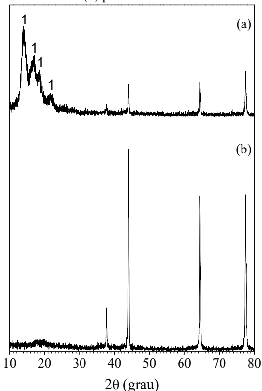
Figura 29 - Difratoograma de raios X da (a) fibra de polipropileno e do (b) porta amostra.
