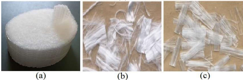
Figura 2 - Cilindro de macrofibras poliméricas (a), fibras de polipropileno monofilamentadas (b) e fibras de polipropileno fibriladas (c).
