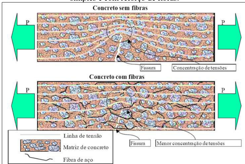
Figura 1 - Esquema de concentração de tensões para um concreto simples e com reforço de fibras.
