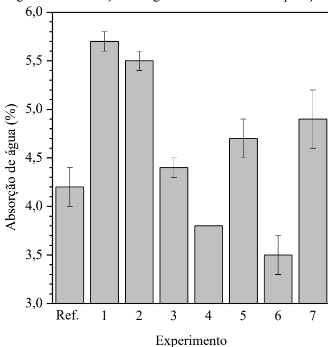
Figura 20 - Absorção de água das diferentes composições.
