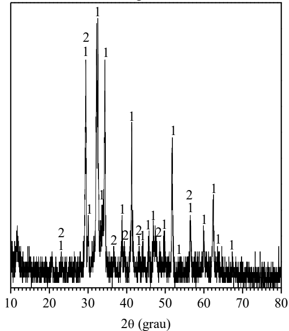
Figura 16 - Difratoograma de raios X do cimento CP V ARI. Onde 1- silicato de alumínio, magnésio e cálcio e 2- calcita.
