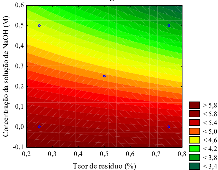
Figura 21 - Superfície de resposta para os resultados de absorção de água.
