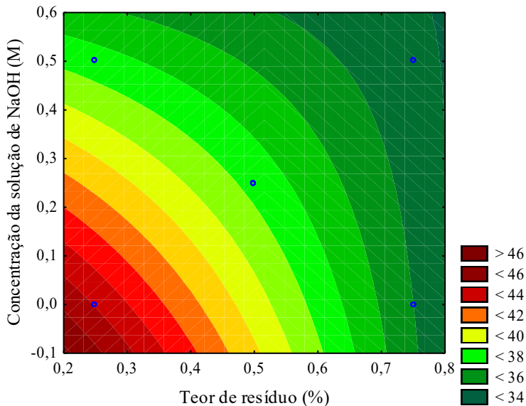
Figura 26 - Superfície de resposta para os resultados de resistência à compressão aos 28 dias.
