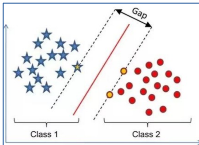
Figura 3 - Método de Máquina de Vetor de Suporte.
