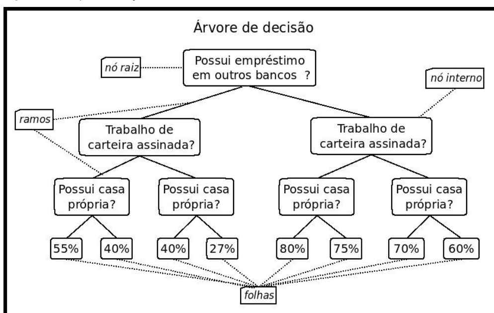
Figura 1 - Representação de uma árvore de Decisão
