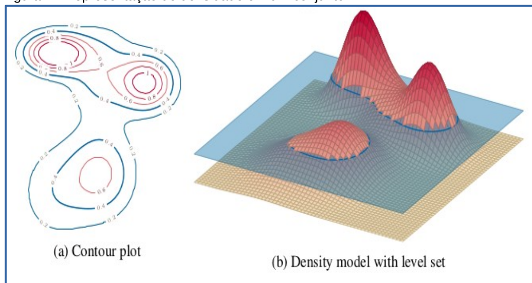
Figura 7 - Representação de densidade em um conjunto
