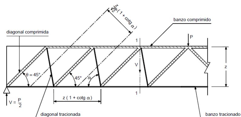
Figura 1 – Viga representada segundo a treliça clássica de Ritter-Mörsch.
